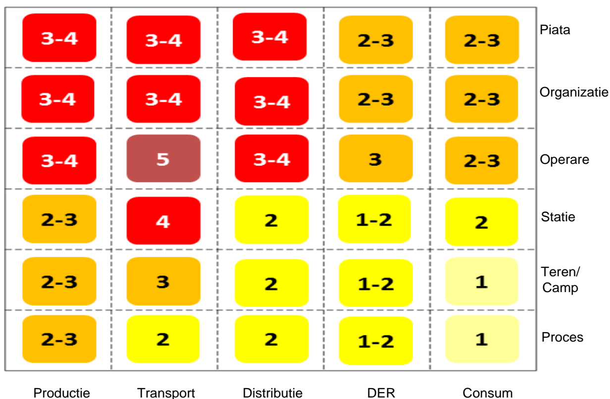
Figura 2 – Maparea nivelurilor de securitate pe arhitectura Smart Grid
